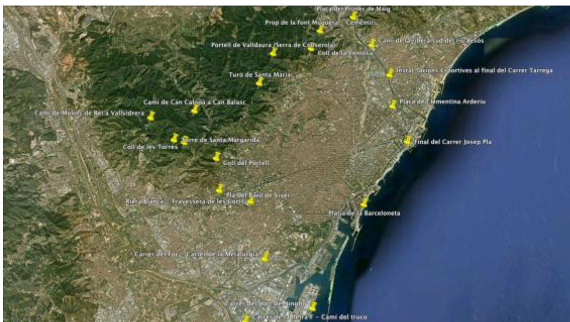
Mapa de las 20 localizaciones de las tomas de sonido del BarcelonaSolÍmit
